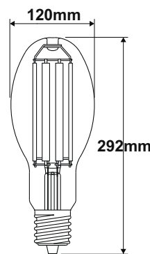
ED120/65W/E40
